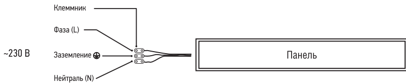
- Рис. 1. Подключение -
